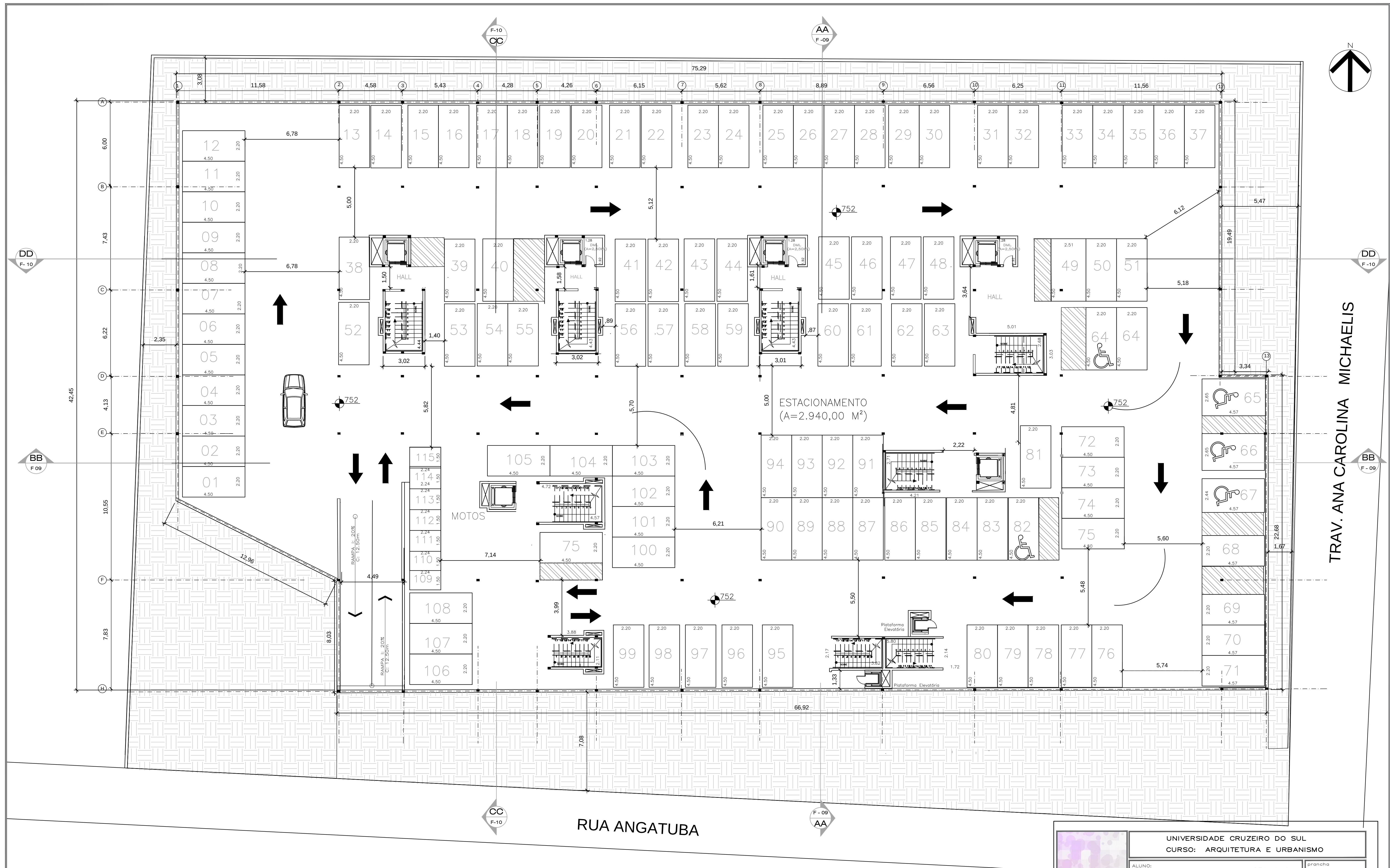
1 PLANTA SUBSOLO - ESTACIONAMENTO ESCALA 1/125
